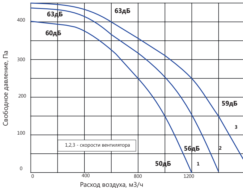
График аэродинамических характеристик установок
