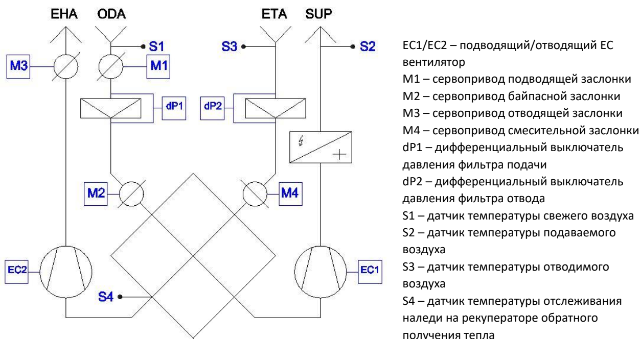
Рис. 14 Система контроля и управления, конфигурация с электрическим нагревателем и смесителем, правый вариант исполнения
