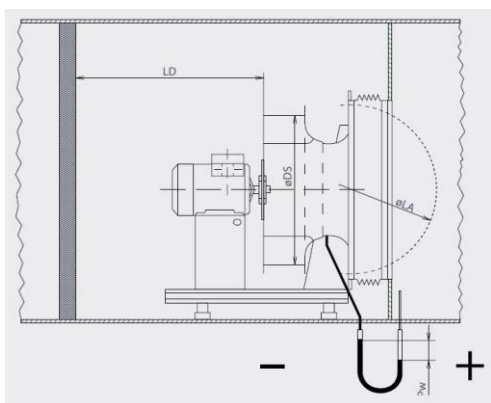
Рис. 10 Присоединение измерительного прибора.
