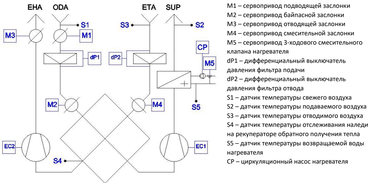
Рис. 13 Система контроля и управления, конфигурация с водяным нагревателем и смесителем, правый вариант исполнения
