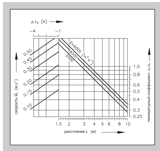
15. VPVM - S 1500
