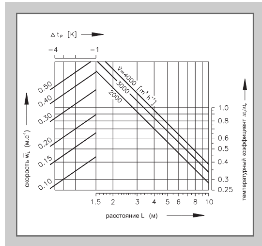
13. VPVM - S 1000
