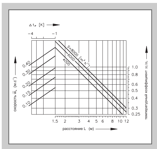
16. VPVM - S 2000
